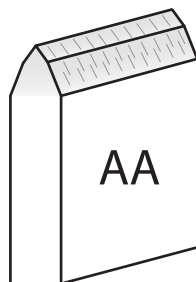
Фасетная центральная заточка
