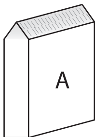
Стандартная двухсторонняя заточка с углом 54^\circ
